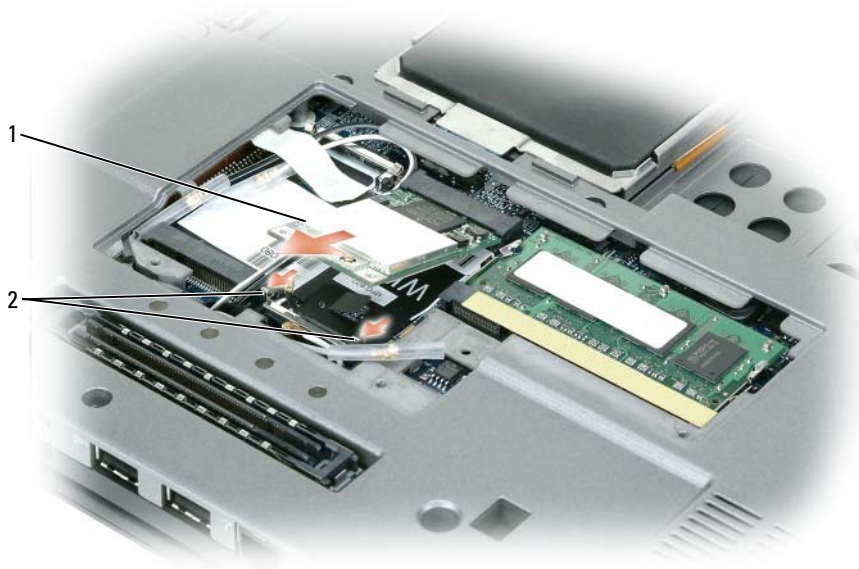
1 WLAN 卡 2 金属固定夹 (2)
