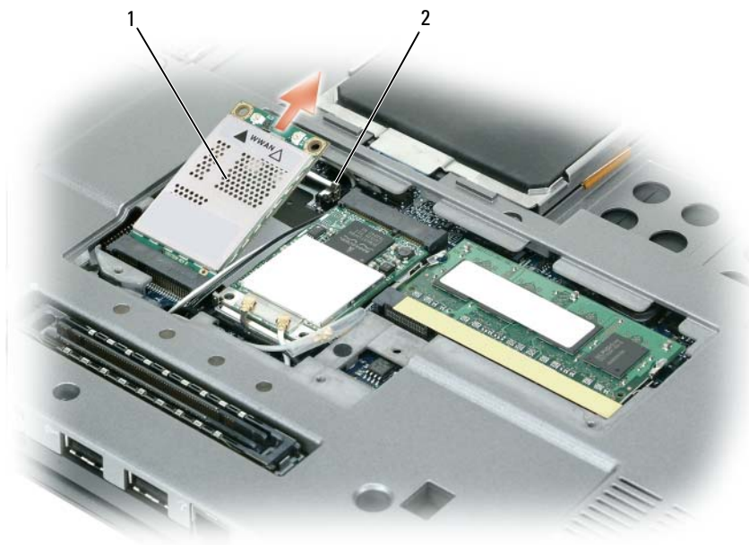
1 移动宽带卡 2 金属固定卡舌 (2)
